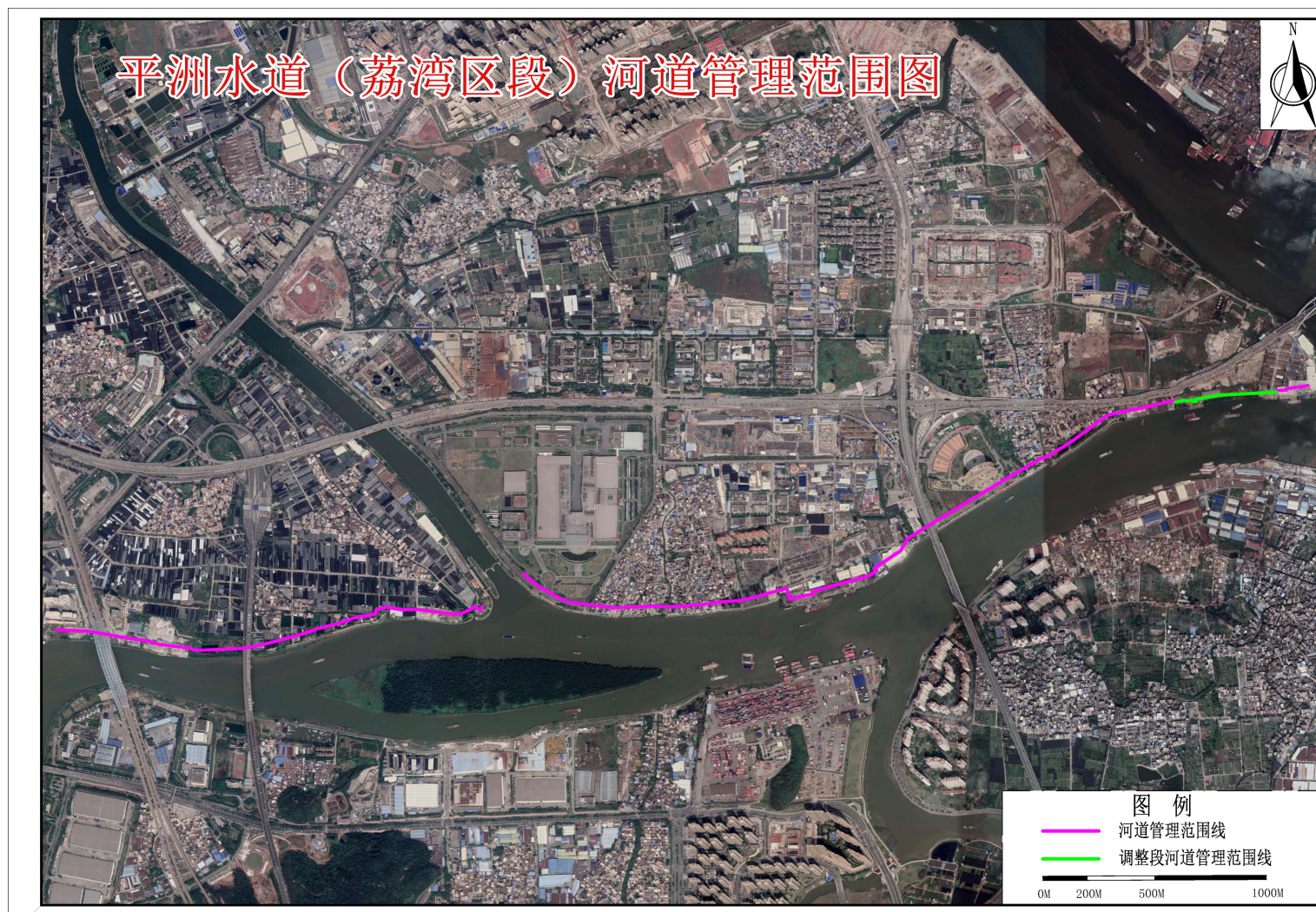
平洲水道（荔湾区段）河道管理范围图
